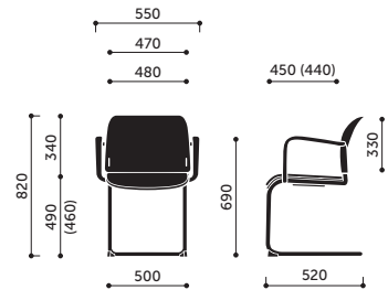
560V / 560V 2P
